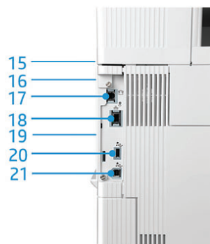
Gros plan des ports d'E/S
